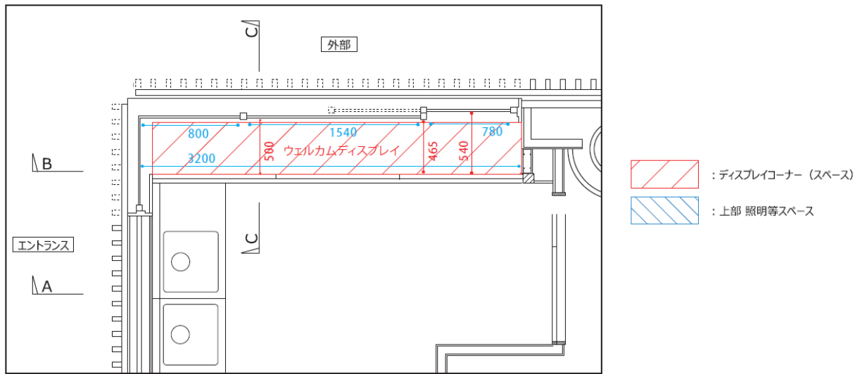
平面詳細図
